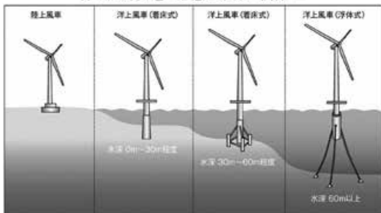
洋上風力発電の形態と水深の関係
